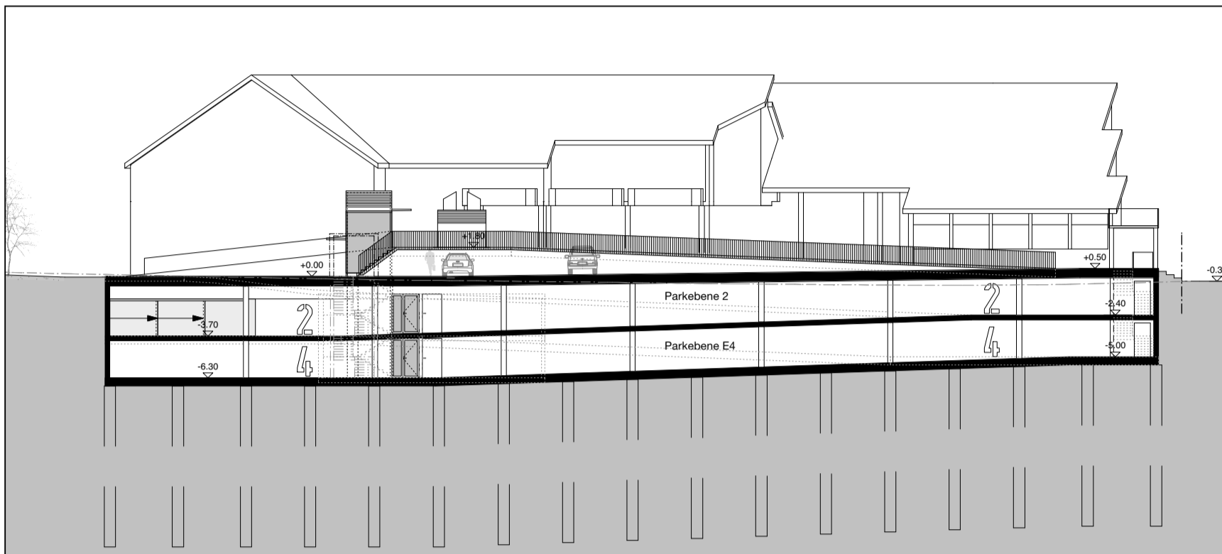
Neue Variante für ein Parkhaus beim Zentrum Monséjour: Durch die Bauweise wird ein Viertel des Volumens eingespart.
